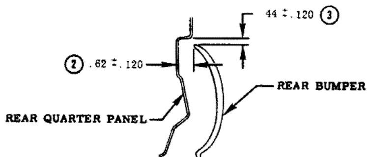
SECTION DD
