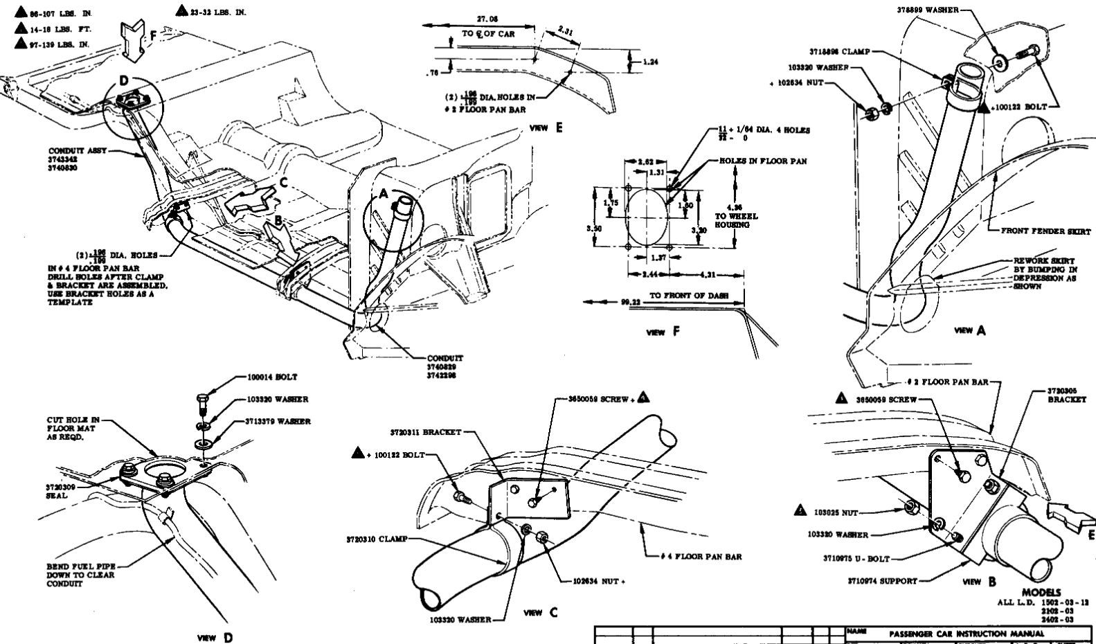
RADIO CONTROL CABLE CONDUIT
